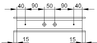
Bohrabstände Deckenmontage
