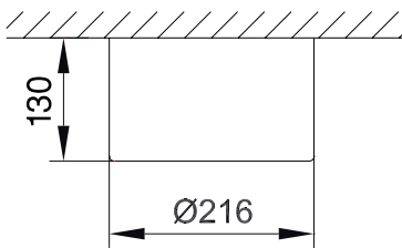
116R3, Deckenmontage
