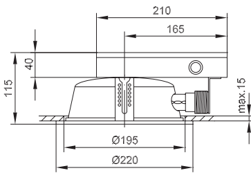
116R2, Hohlraumeinbau
