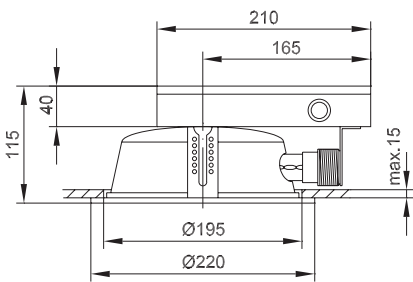
216R2, Hohlraumeinbau
