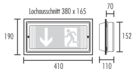
208W, Einbaumontage
