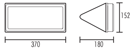
208D, Deckenmontage
