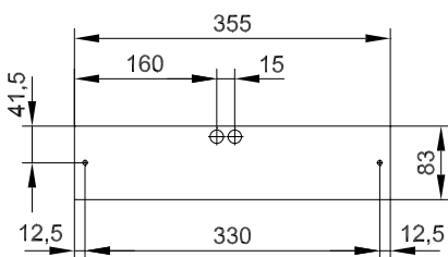
Bohrabstände
